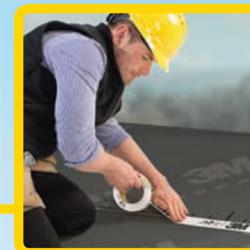
Герметизация и защита от ветра перекрытий и гидроизоляции крыши: 3M™ FAST-G 8068E
