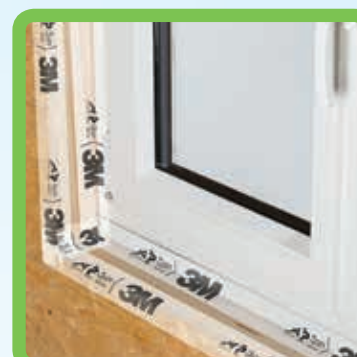
Быстрая герметизация окон и дверей благодаря разделенному бумажному защитному лайнеру: 3M™ FAST-F 8067E
