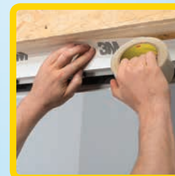
Герметизация пароизоляции на мансардных окнах: 3M™ FAST-G 8068E
